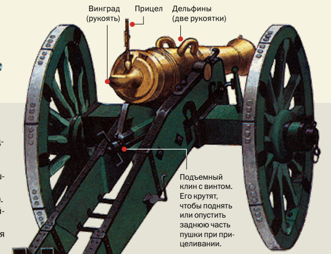
Калибр.....120 мм Длина ствола.....1,2 м Вес орудия.....668,3 кг
